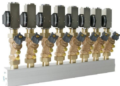
Фото - блок клапанов VB2-020GA8, с клапанами и датчиком потока M101
